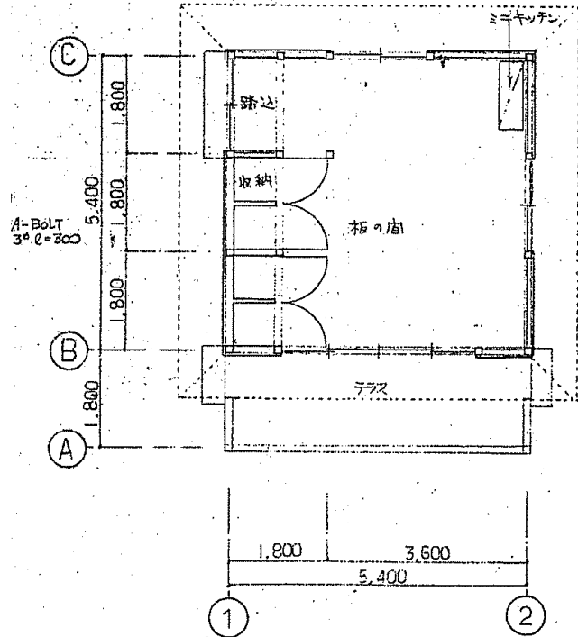
1階平面図
