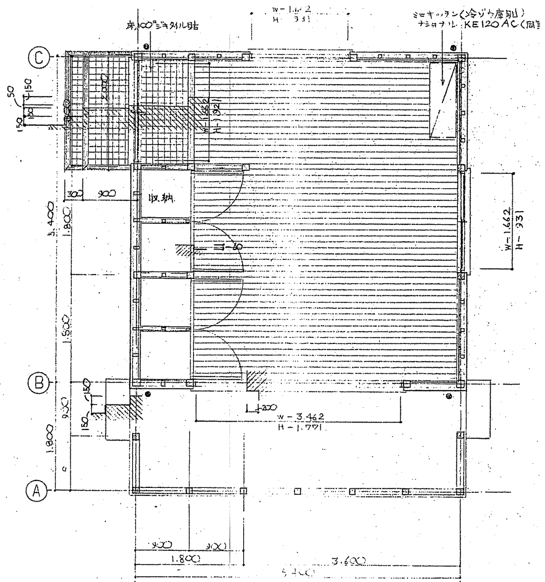
1階平面詳細図
